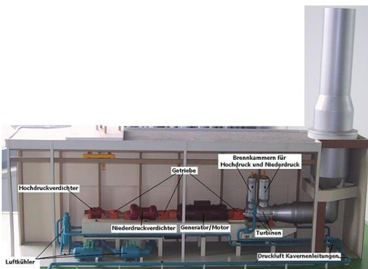
Abbildung 3 Druckluftspeicherkraftwerks Modell 10
