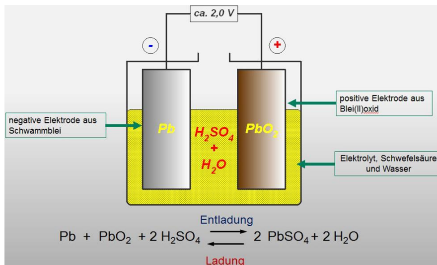
Abbildung 1 Schematische Darstellung vom Aufbau eines Bleiakкумуляtors und der chemische Reaktionen beim Laden und Entladen. 1
