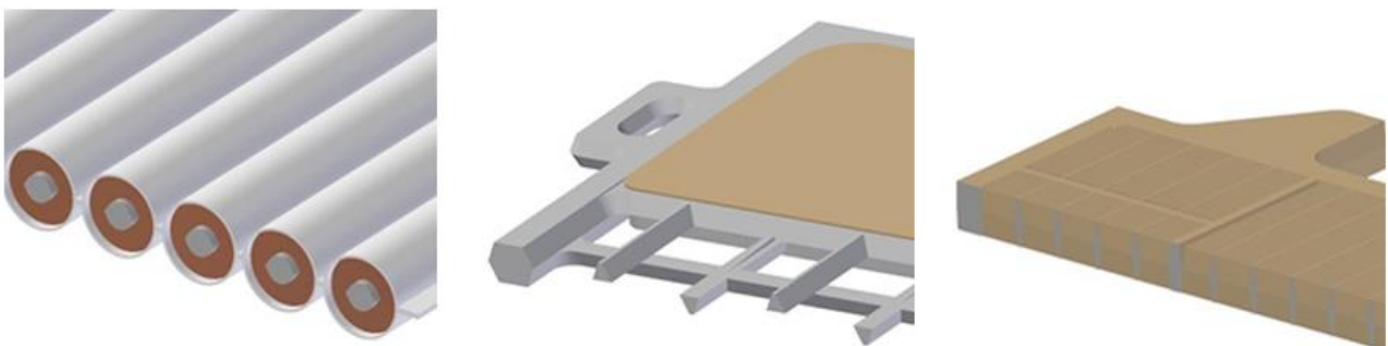
Abbildung 3: Von links nach rechts: Panzerplattenbatterie, Gitterplattenbatterie, Großoberflächenbatterie
