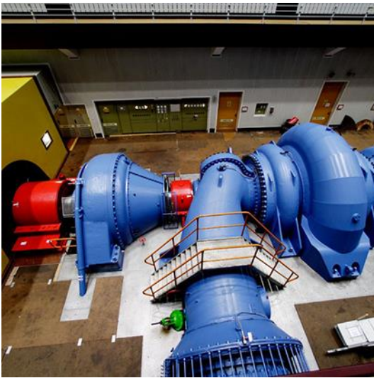
Abbildung 2: Pumpe des PSW Wehr der Schluchseewerk AG
